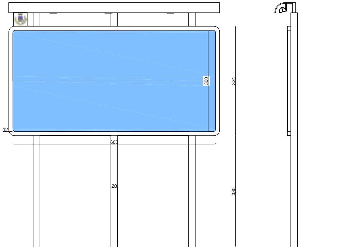
PROSPETTO FRONTALE
