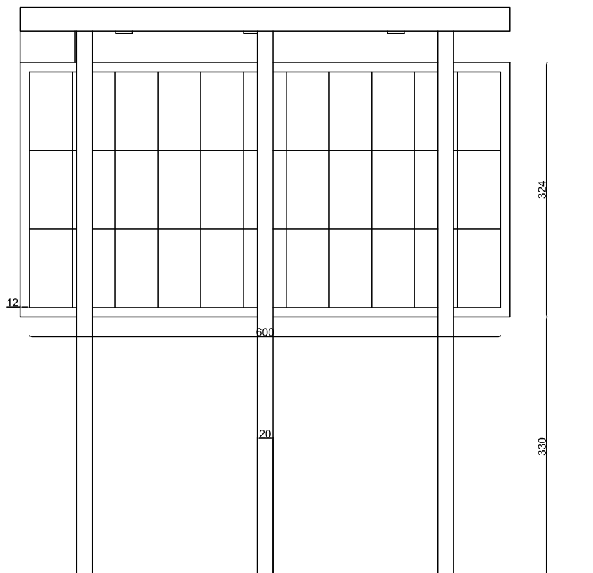
PROSPETTO RETRO
